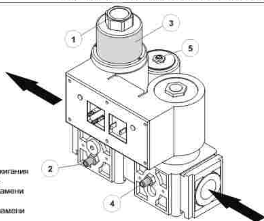
Рис. 9.3 Электроклапан Eolo 115-140
