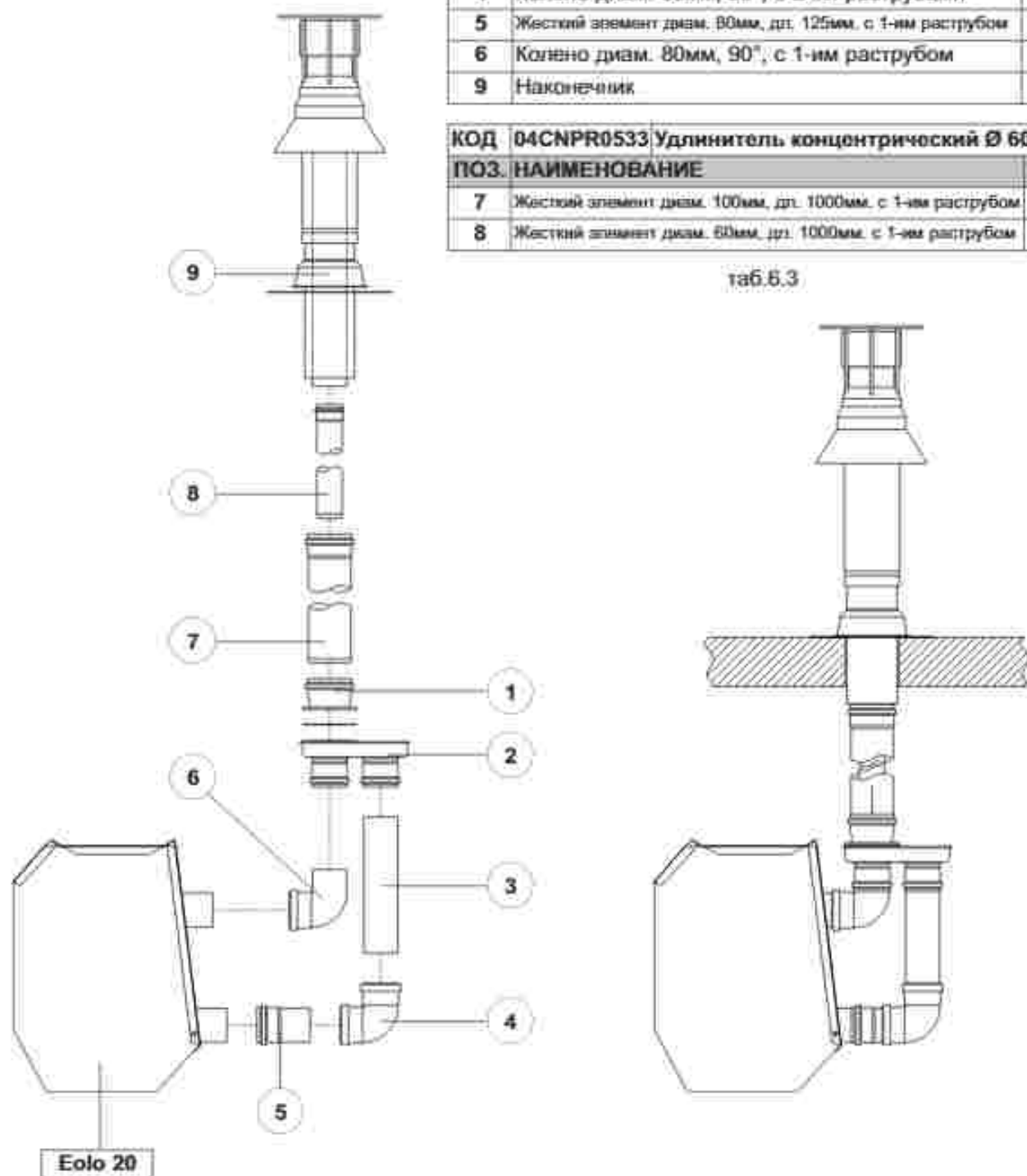
Рис. 6.1 Пример устройства саосного дымохода-воздуховода аппарата «EOLIO 20» через крышу
