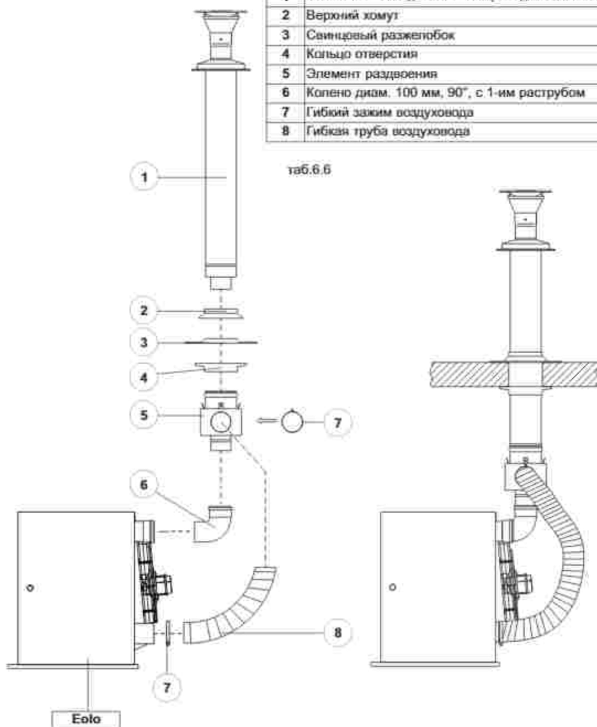
Рис. 6.4 Пример устройства соосного дымохода-воздуховода аппаратов "EOLO 30-50-70-90" через крышу
