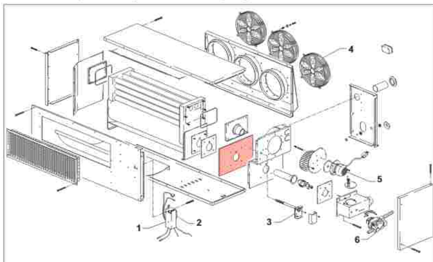
Рис. 3.9 Деталировка Eolo90AE
