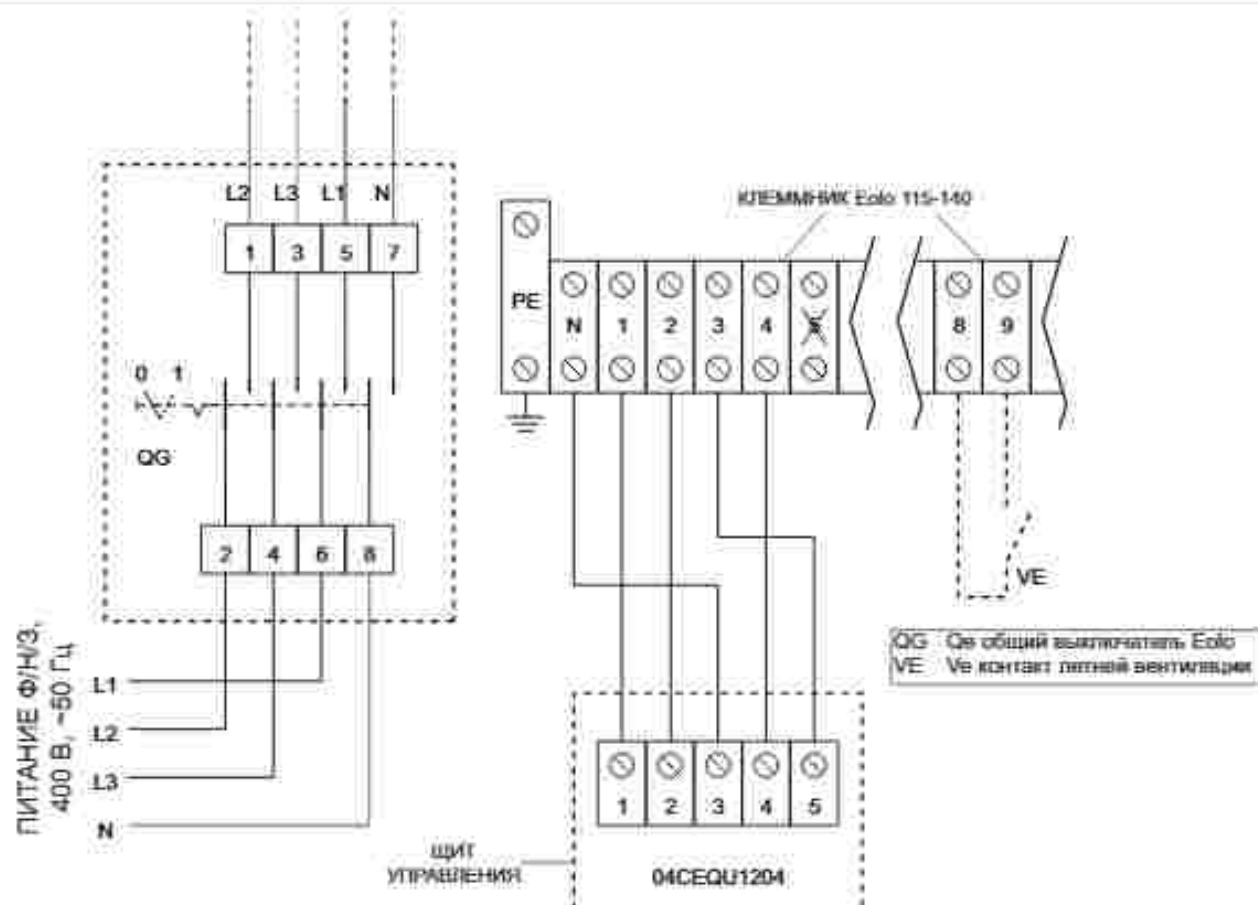
Рис.В.4 Схема подключения к щитам для Еolo 115-140 мод. 04CEQU1204
