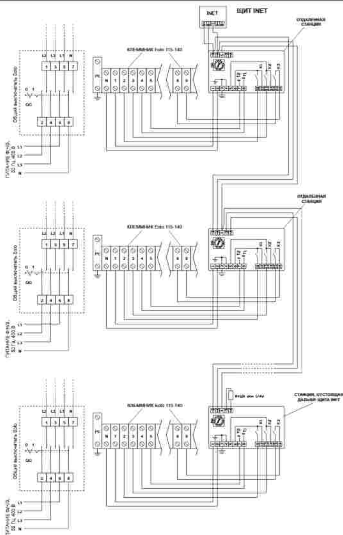
Рис. 8.7 Схема подключения к щитам Eolo 115-140 типа «INET»
