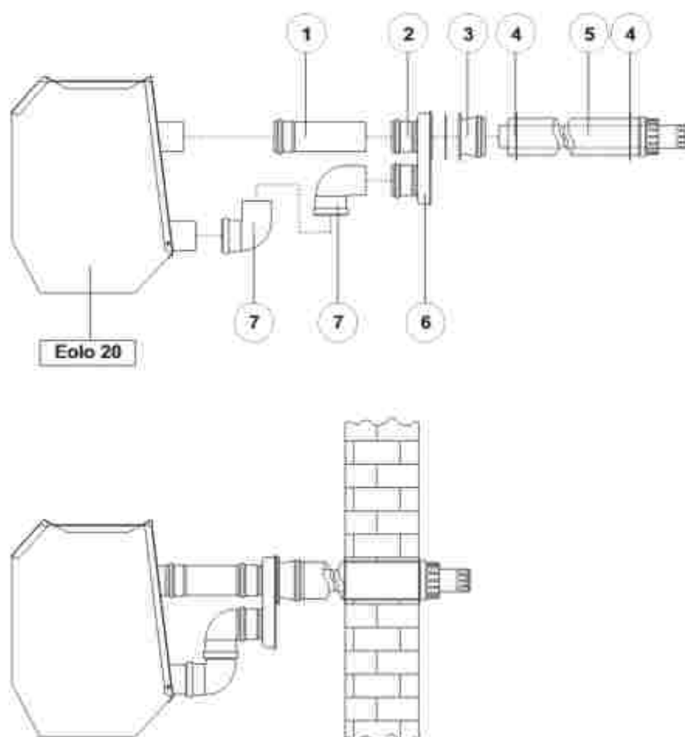
Рис. 6.2 Пример устройства соосного дымохода-воздуховода аппарата "EOLO 20" через стену
