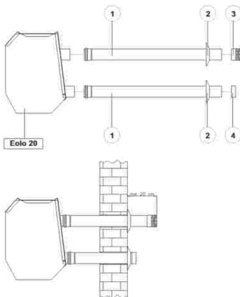
Рис. 6.3 Пример устройства дымохода и воздуховода аппарата «Еоло 20» через стену
