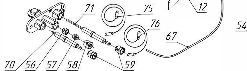
Состав пилотной горелки (поз. 35)
