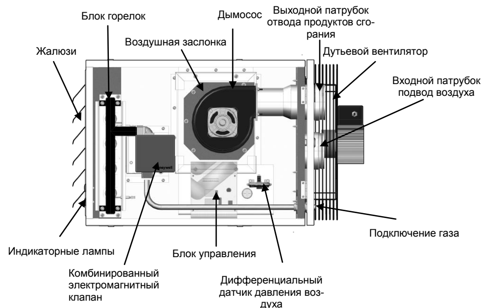
Рис 2.: Основные узлы воздушонагревателя
