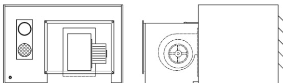
Рис 5.: Воздухонагреватели с центробежным вентилятором
