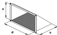
Наружный воздухозаборник с защитной решеткой (KLM...)
