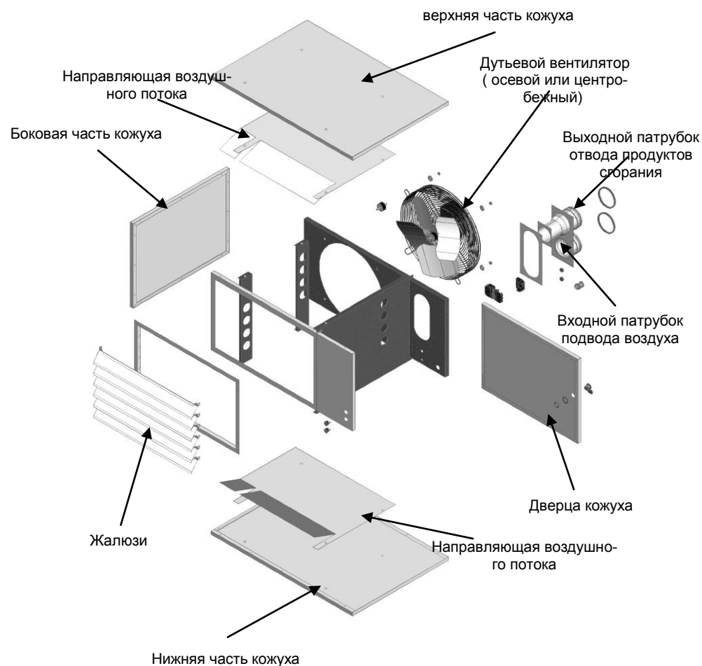
Рис 1/б.: Внешнее устройство воздушонагревателя
